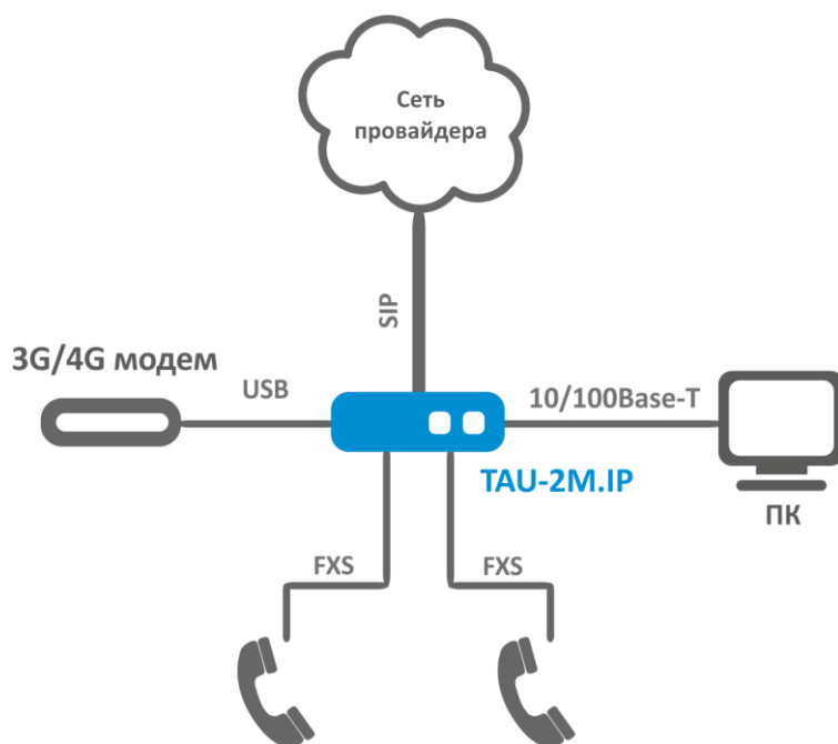
Рисунок 1 – Функциональная схема использования TAU-2M.IP
