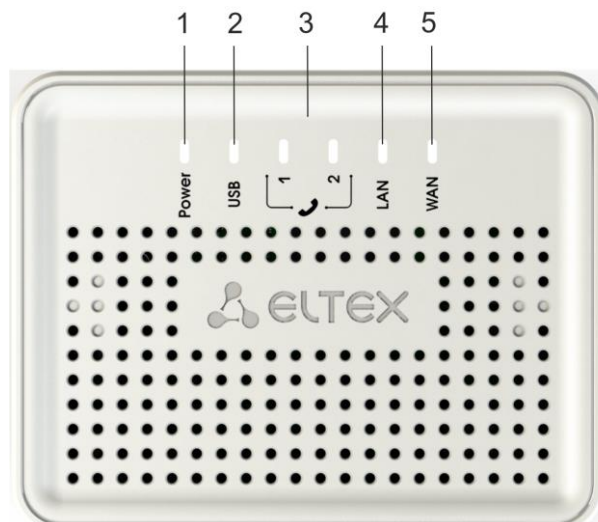
Рисунок 4 – Внешний вид верхней панели TAU-2M.IP
