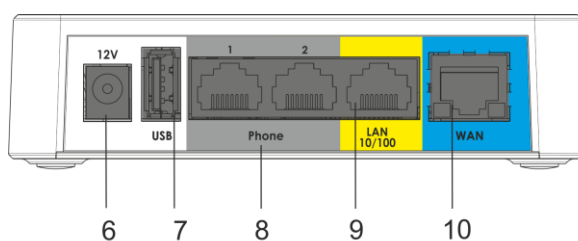
Рисунок 5 – Внешний вид задней панели TAU-2M.IP
